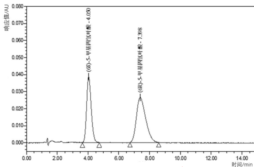
图C.3 (6S)-5-甲基四氢叶酸和(6R)-5-甲基四氢叶酸参考液相色谱图
