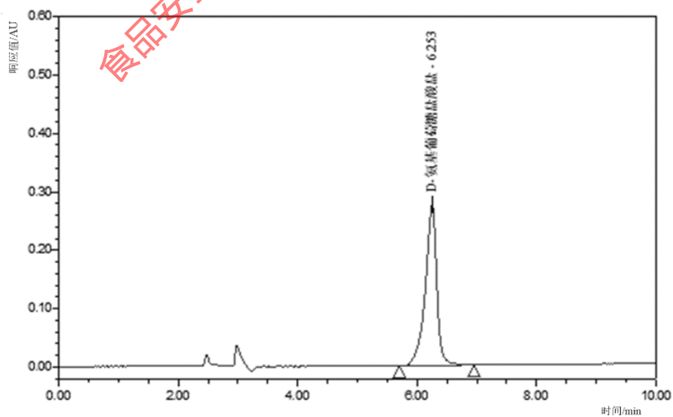
图C.2 氨基葡萄糖盐酸盐参考液相色谱图
