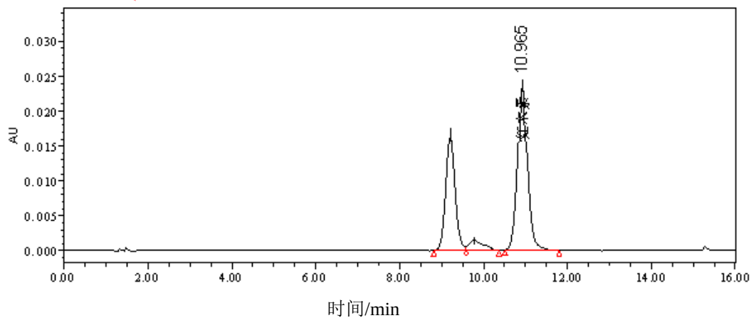
图A.3 含顺、反构型的红木素溶液的液相色谱图
