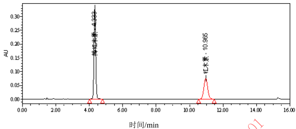
图A.1 顺式降红木素和顺式红木素标准溶液液相色谱图
